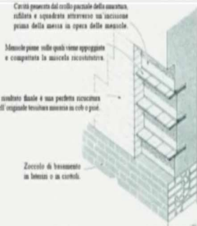
Metodo per la ricostruzione della muratura degradata in bauge o pisé.
